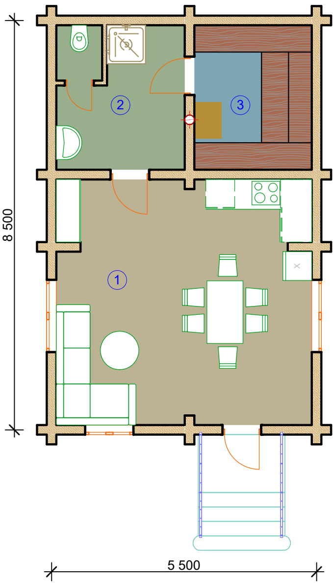
Експлікація приміщень 1 поверх
