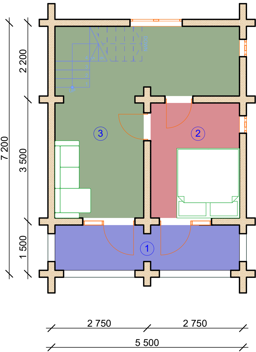
Експлікація приміщень 2 поверх
