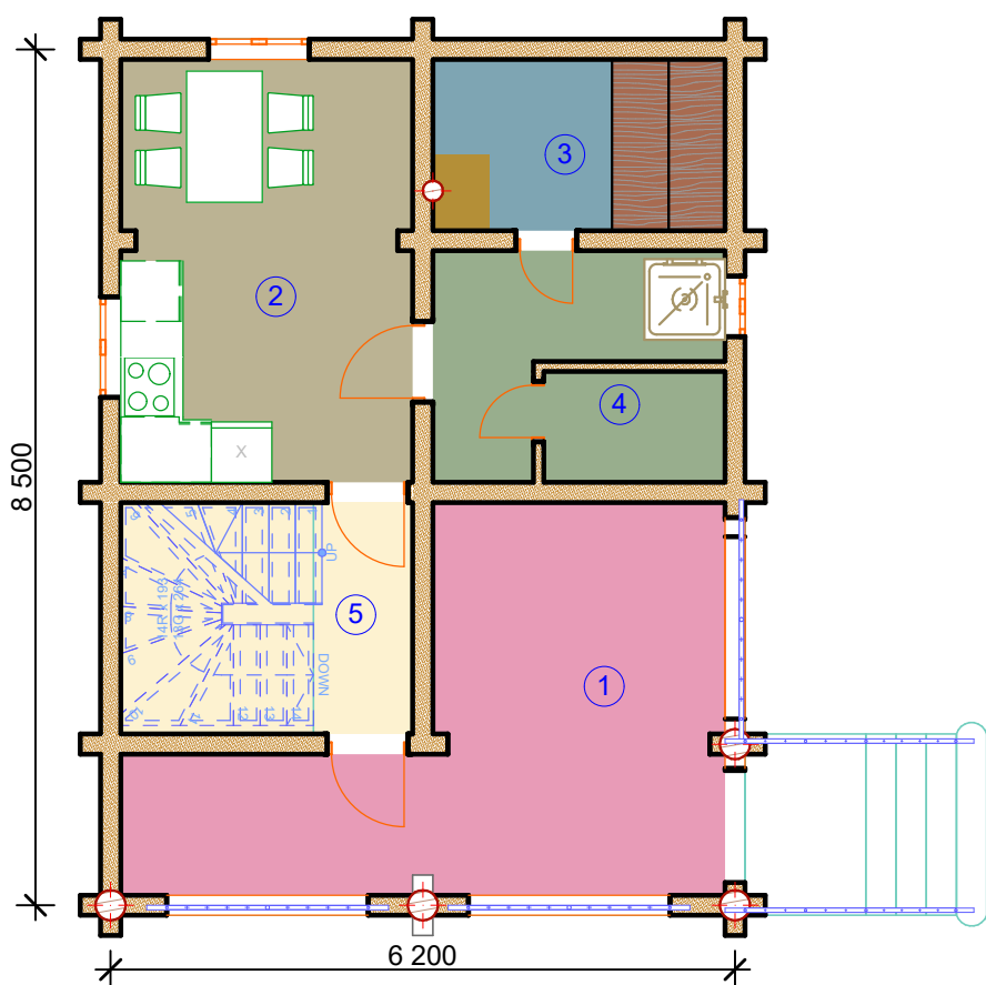
Експлікація приміщень 1 поверх
