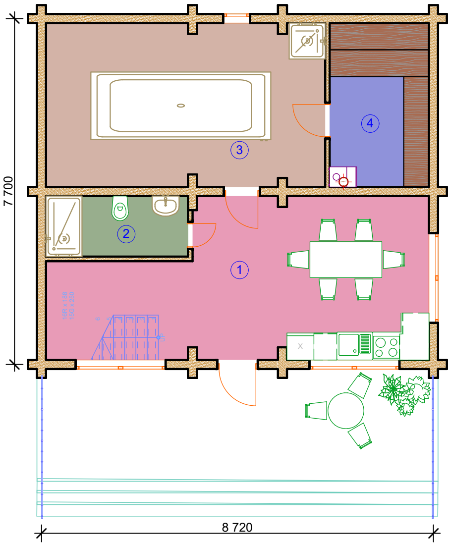
Експлікація приміщень 1 поверх
