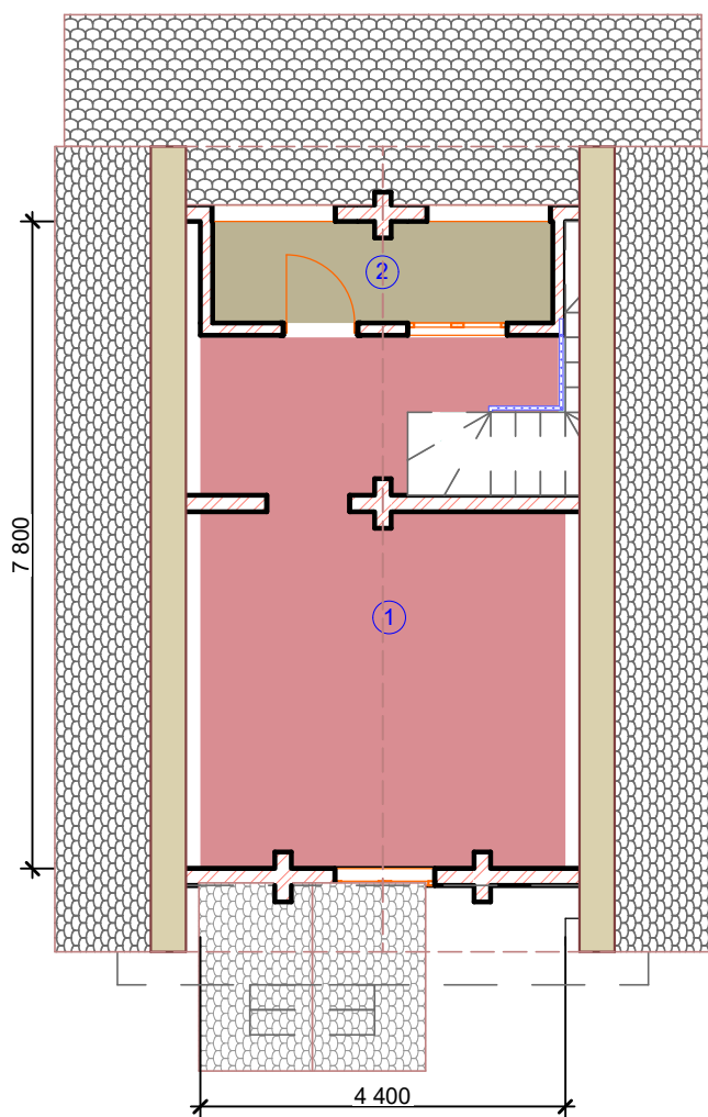
Експликація приміщень 2 етаж
