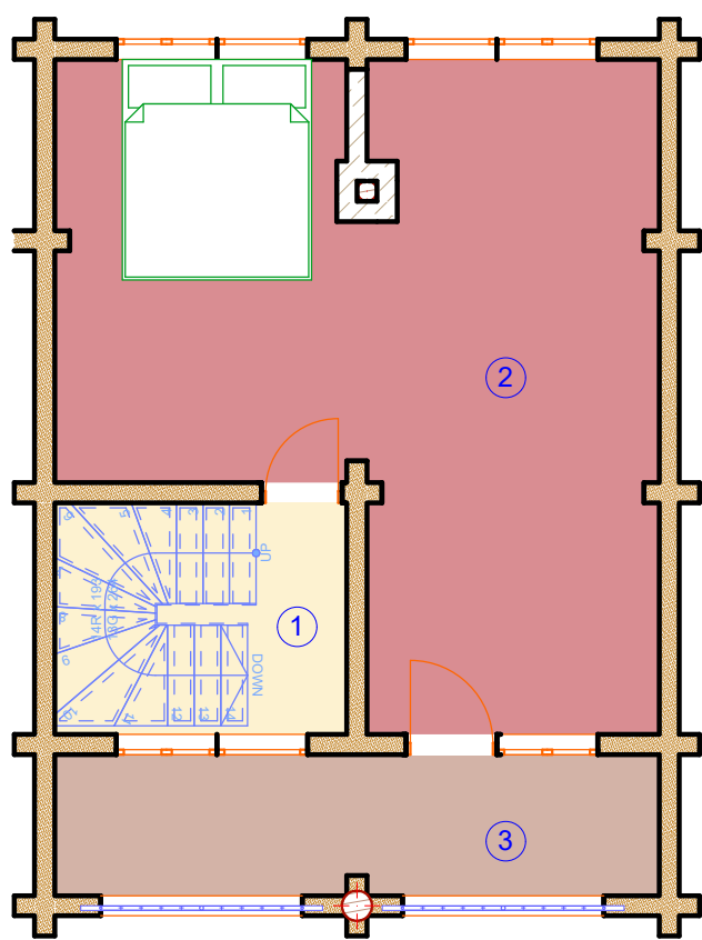
Експлікація приміщень 2 поверх
