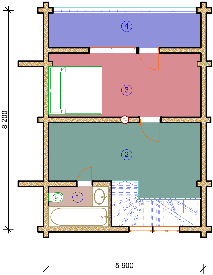
Експлікація приміщень 2 поверх
