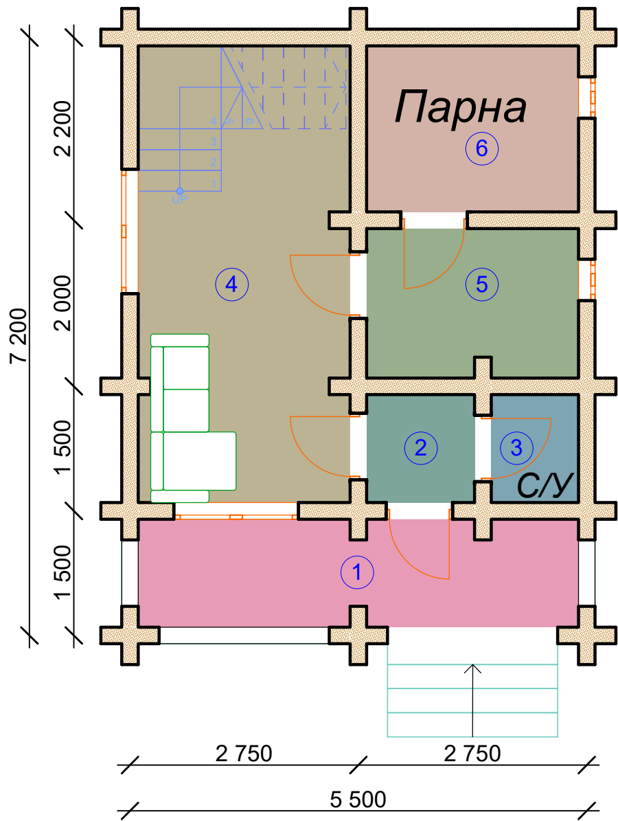
Експлікація приміщень 1 поверх
