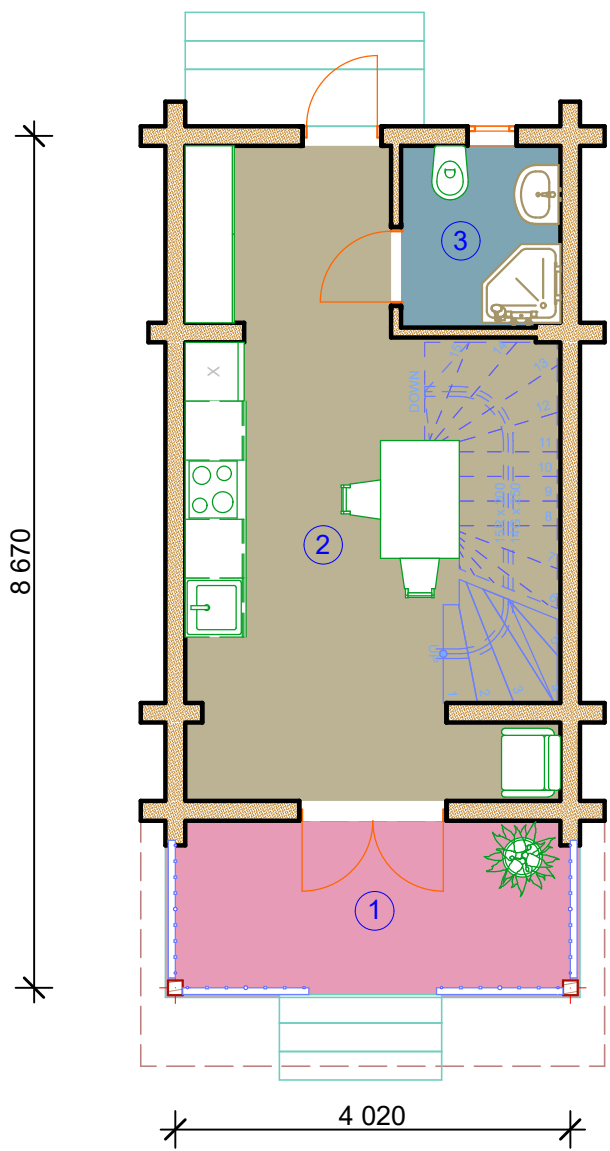
Експлікація приміщень 1 поверх
