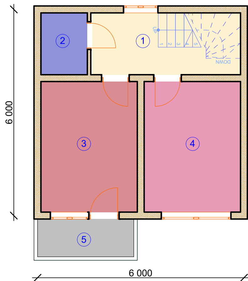
Експлікація приміщень 2 поверх
