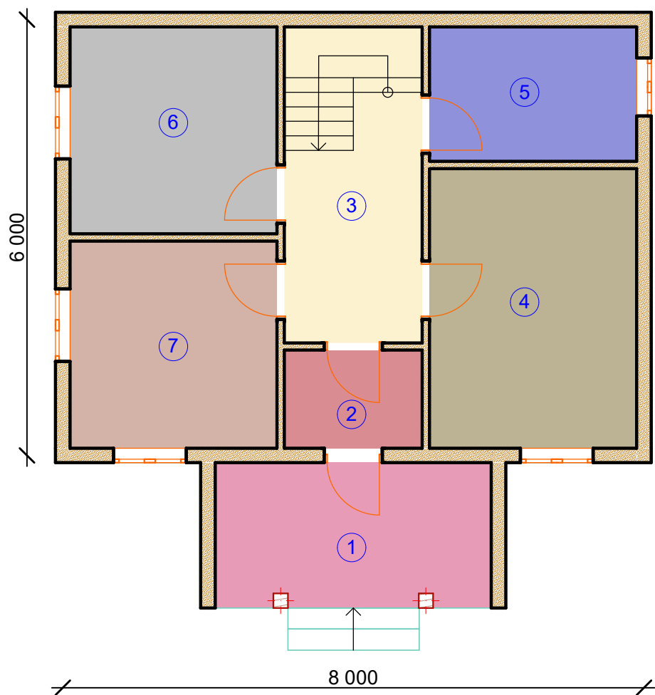
Експлікація приміщень 1 поверх
